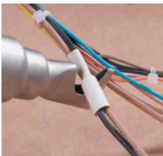
Skupljanje termogenih navlaka
