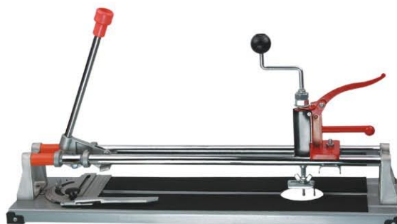
Rezač keramičkih pločica sa bušačem rupa
